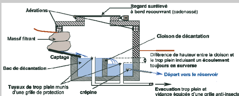
Ci-dessus : Schéma de principe d'un captage, bac décantation et réservoir
