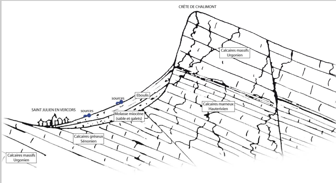
Ci-dessus : Coupe géologique schématique (La zone de chevauchement n'est pas détaillée)
